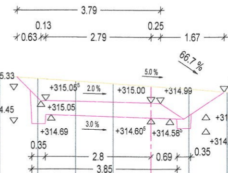
Staničení : 0+020.00
