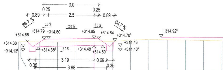
Staničení : 0+005.00
