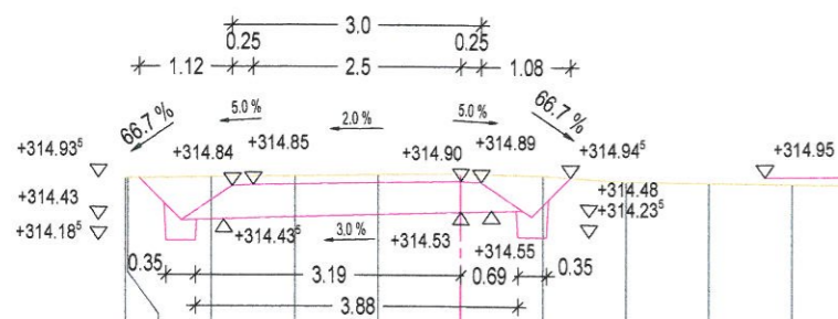
Staničení : 0+010.00
