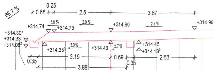
Staničení : 0+000.00
